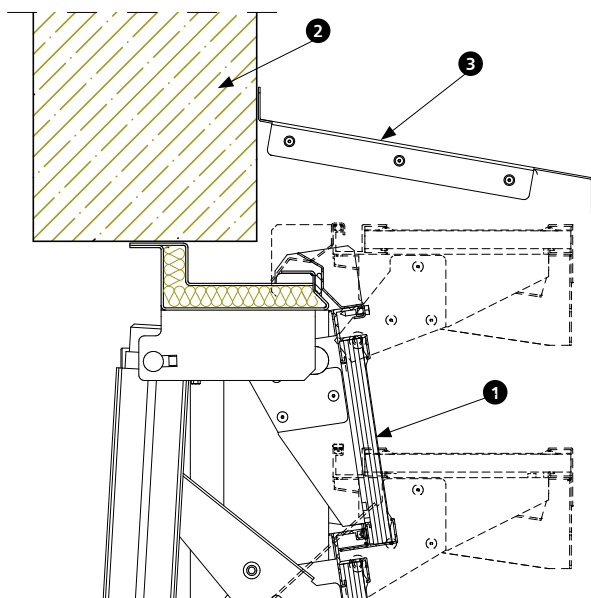
Rys. 14 Montaż kłapy żaluzjowej bezpośrednio do ściany (fasady)
