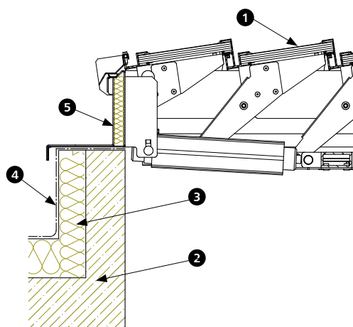
Rys. 9 Montaż kłapy żaluzjowej z podstawą nakładkową ocieploną na dachu, na istniejącym cokole
