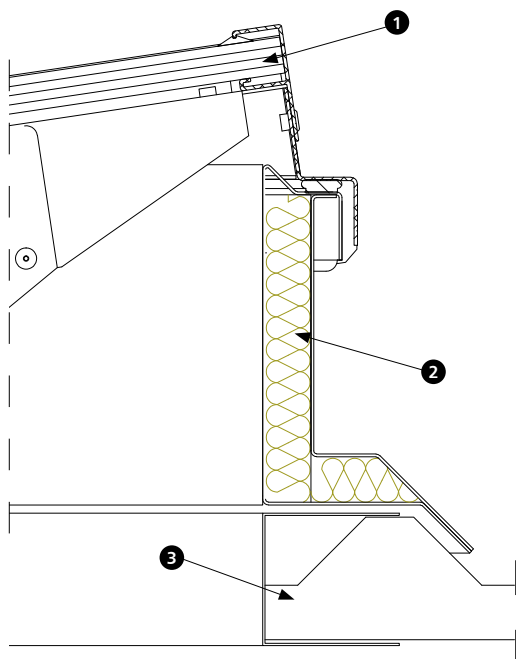
Rys. 11 Montaż kłapy żaluzjowej na dachu systemowym krytym blachą
