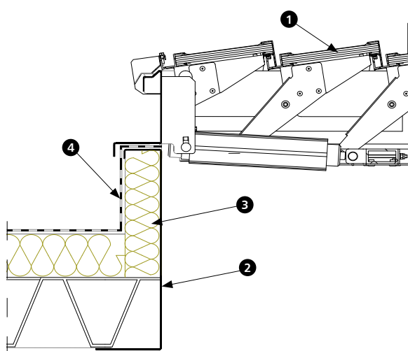
Rys. 10 Montaż kłapy żaluzjowej z podstawą nakładkową nieocieploną na dachu, na cokole stalowym
