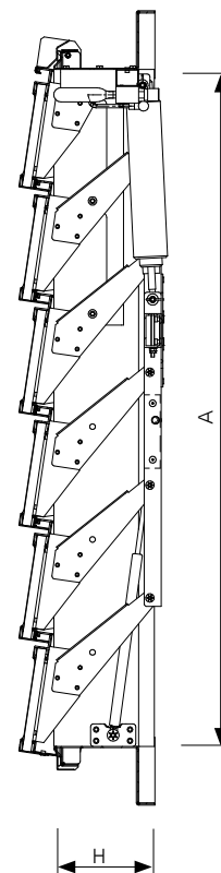
Rys. 8 Przekrój A-A przez klapę żaluzjową napowietrzającą mcr LAM-N w pozycji zamkniętej, (montaż w fasadzie)
