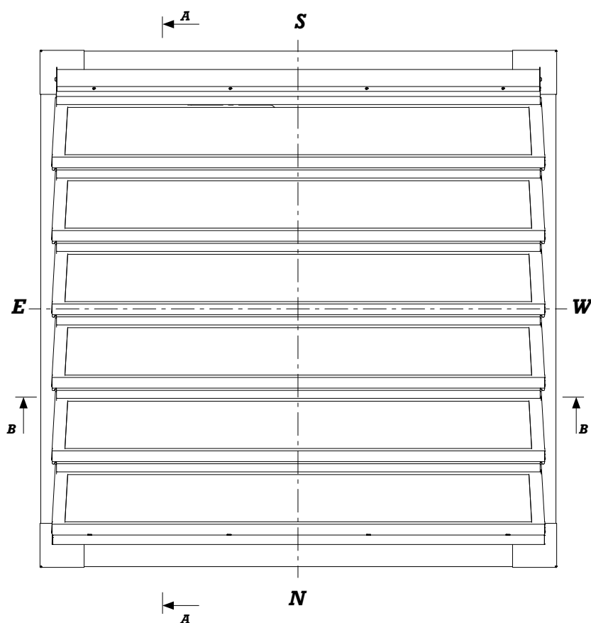
Rys. 7 Widok z góry kłapy żaluzjowej napowietrzającej mcr LAM-N w pozycji zamkniętej
