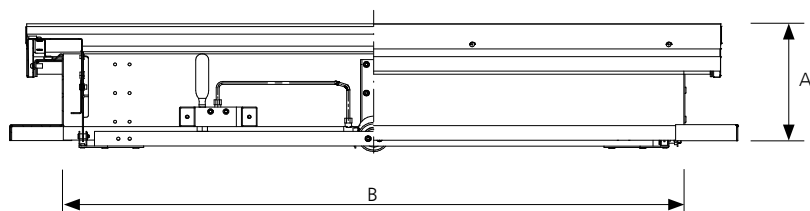
Rys. 6 Przekrój B-B przez klapę żaluzjową napowietrzającą mcr LAM-N w pozycji zamkniętej (montaż w fasadzie)
