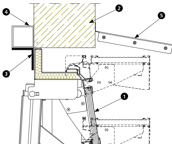
Rys. 12 Montaż kłapy żaluzjowej w ścianie (fasadzie) za pomocą dodatkowego profilu stalowego
