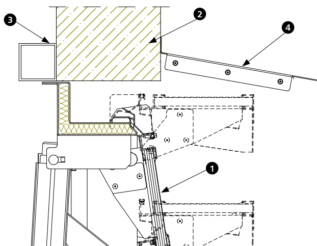
Rys. 13 Montaż kłapy żaluzjowej w ścianie (fasadzie) do konstrukcji wsporczej
