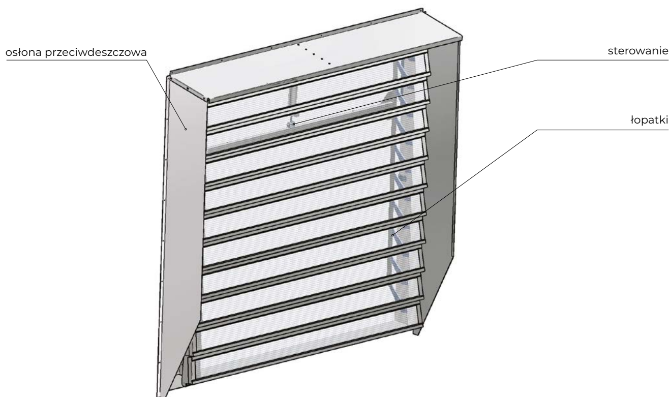
Rys. 5 Budowa kłapy żaluzyjowej napowietrzającej mcr LAM-N wyposażonej w osłonę przeciwdeszczową
