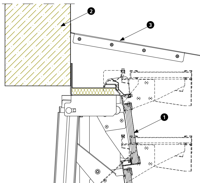
Rys. 15 Montaż kłapy żaluzjowej bezpośrednio do ściany (fasady) od strony zewnętrznej
